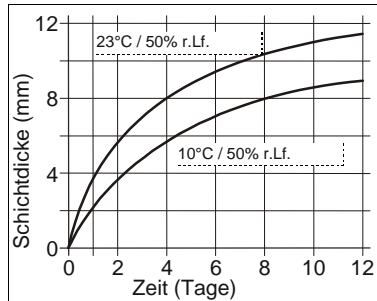
Diagramm 1: Durchhärtungsgeschwindigkeit für Sikaflex®-295 UV
