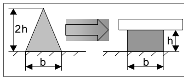
Abbildung 1: Empfohlener Klebstoffauftrag
